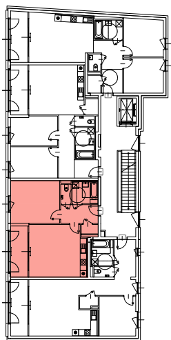
ÜBERSICHT - BLOCK 1 - 4.OG - TOP 1/11
